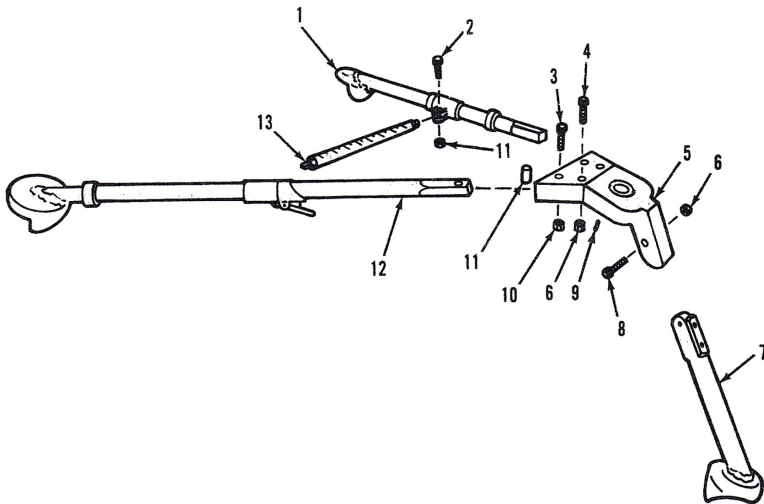
ภาพที่ 30 ขาหยังปืนกล M122 (องค์ประกอบหลัก)
