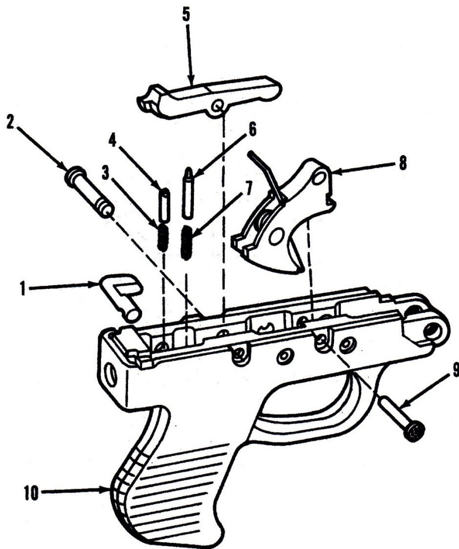
ภาพที่ 9 ด้ามปืนและชุดเครื่องลั่นไก (เฉพาะ M60)
