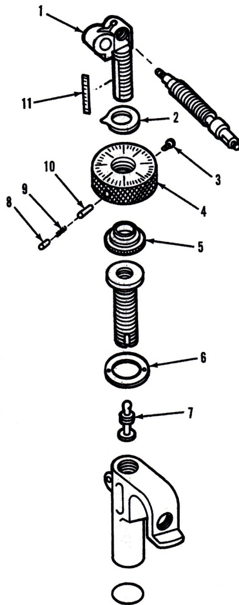
ภาพที่ 32 ชุดกลไกให้มุมทางทิศและทางสูง (ชุดให้มุมทางสูง)
