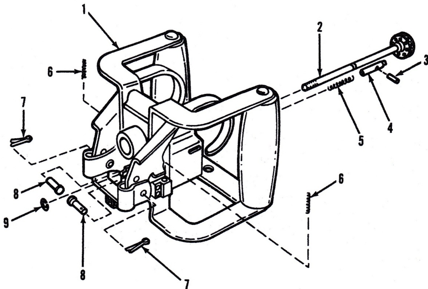
ภาพที่ 6 ต่อมปั๊มและชุดเครื่องกลั่นไถ (เฉพาะ M60D)
