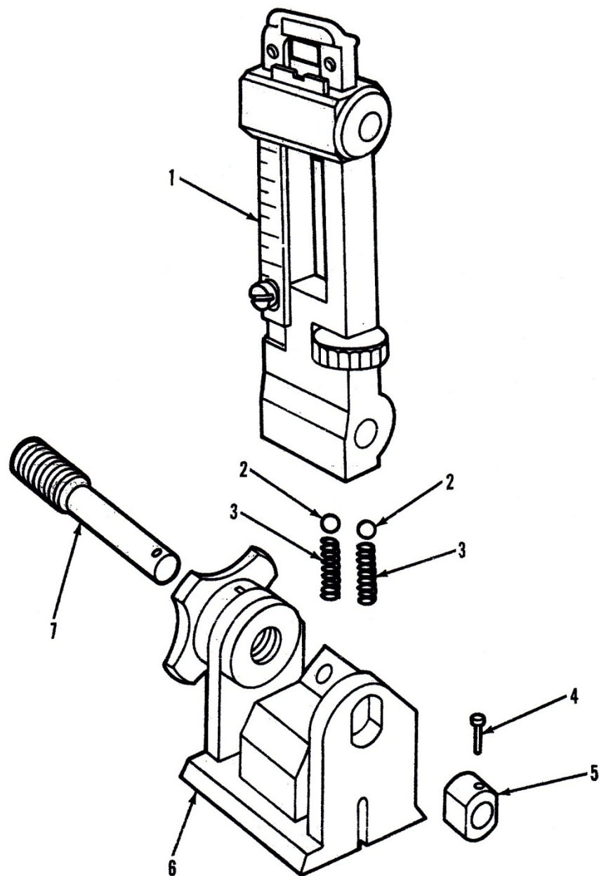
ภาพที่ 23 ศูนย์หลัง (เฉพาะ M60)
