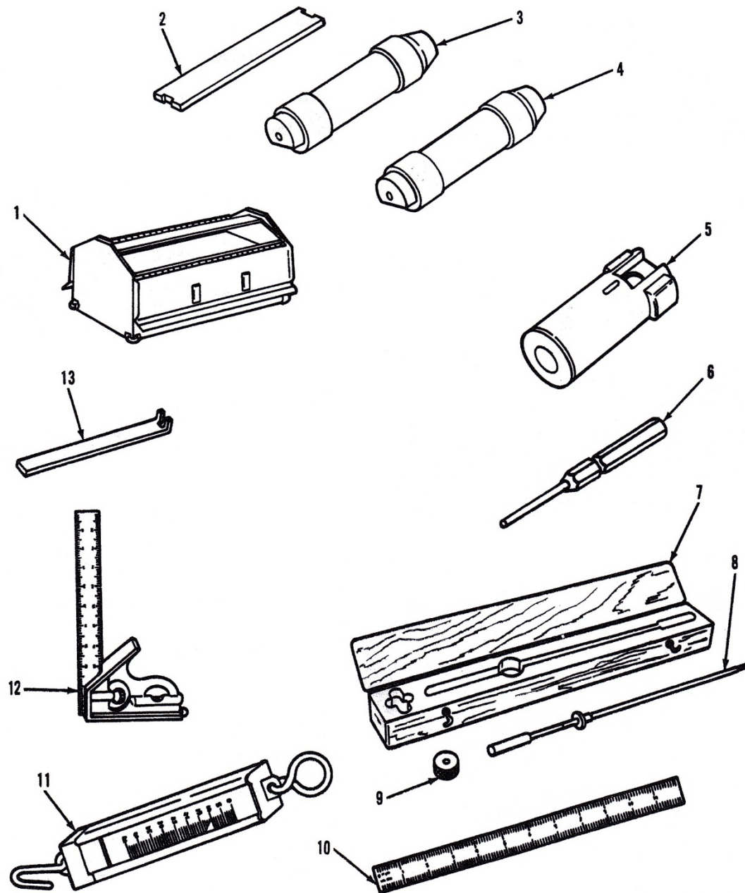
ภาพที่ 36 เครื่องมือพิเศษ
