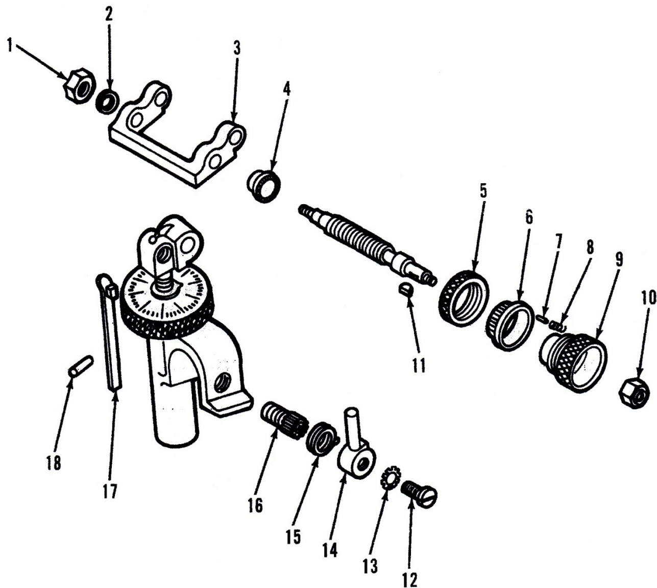
ภาพที่ 31 ชุดกลไกให้มุมทางทิศและทางสูง (ชุดขायึดและให้มุมทางทิศ)
