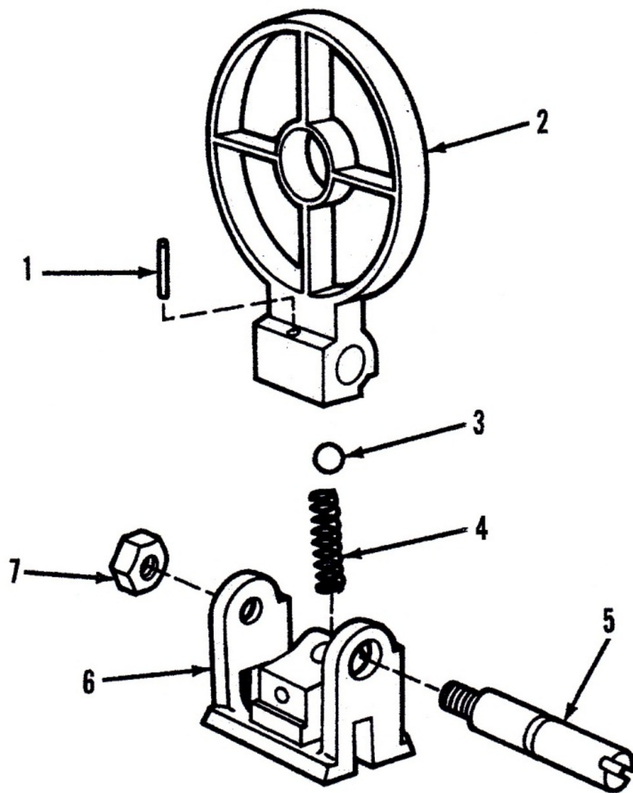
ภาพที่ 25 ศูนย์หลัง (เฉพาะ M60D)
