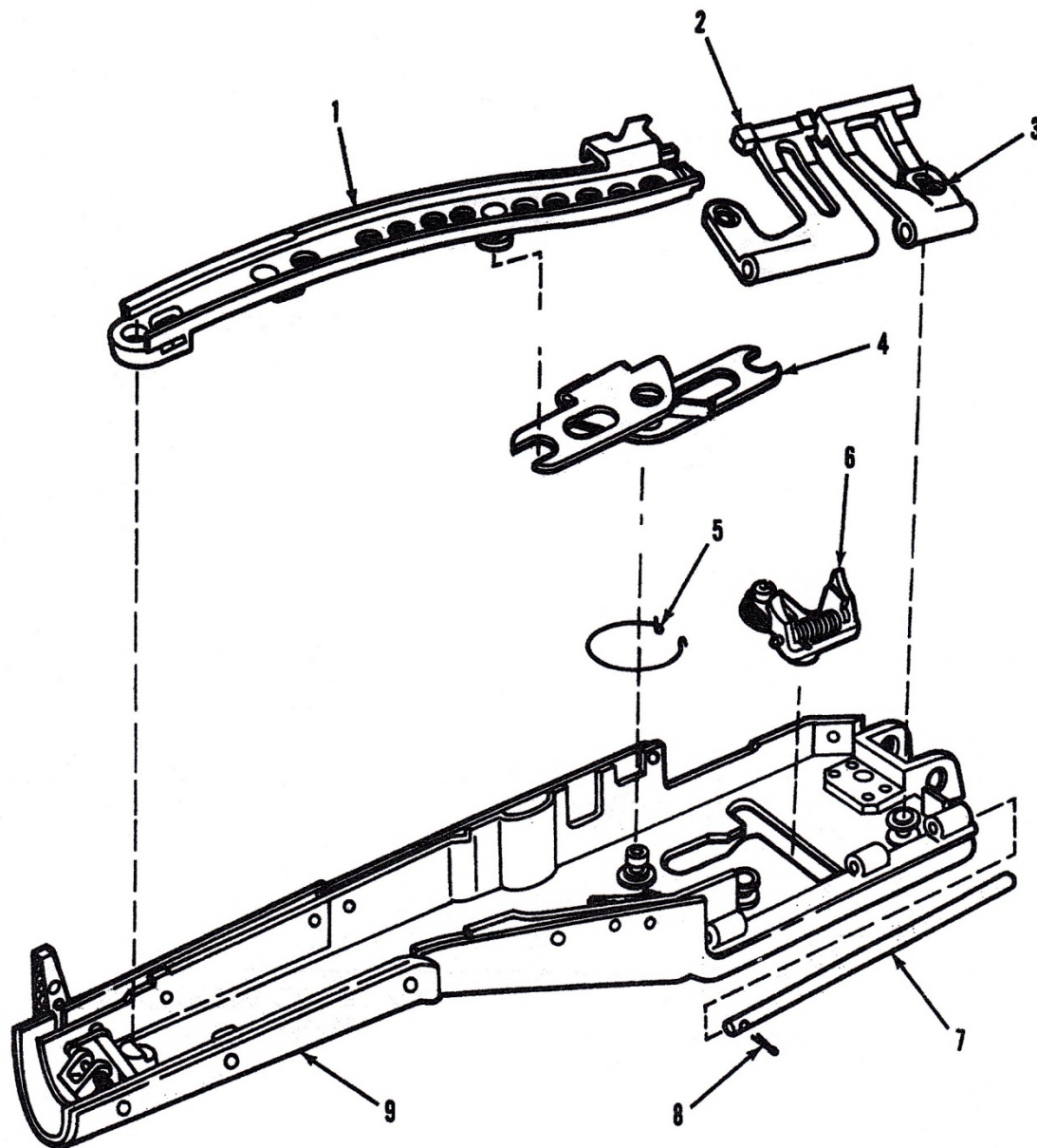
ภาพที่ 15 ฝาปิดห้องลูกเลื่อน และชุดคันเลื่อนสายกระสุน
