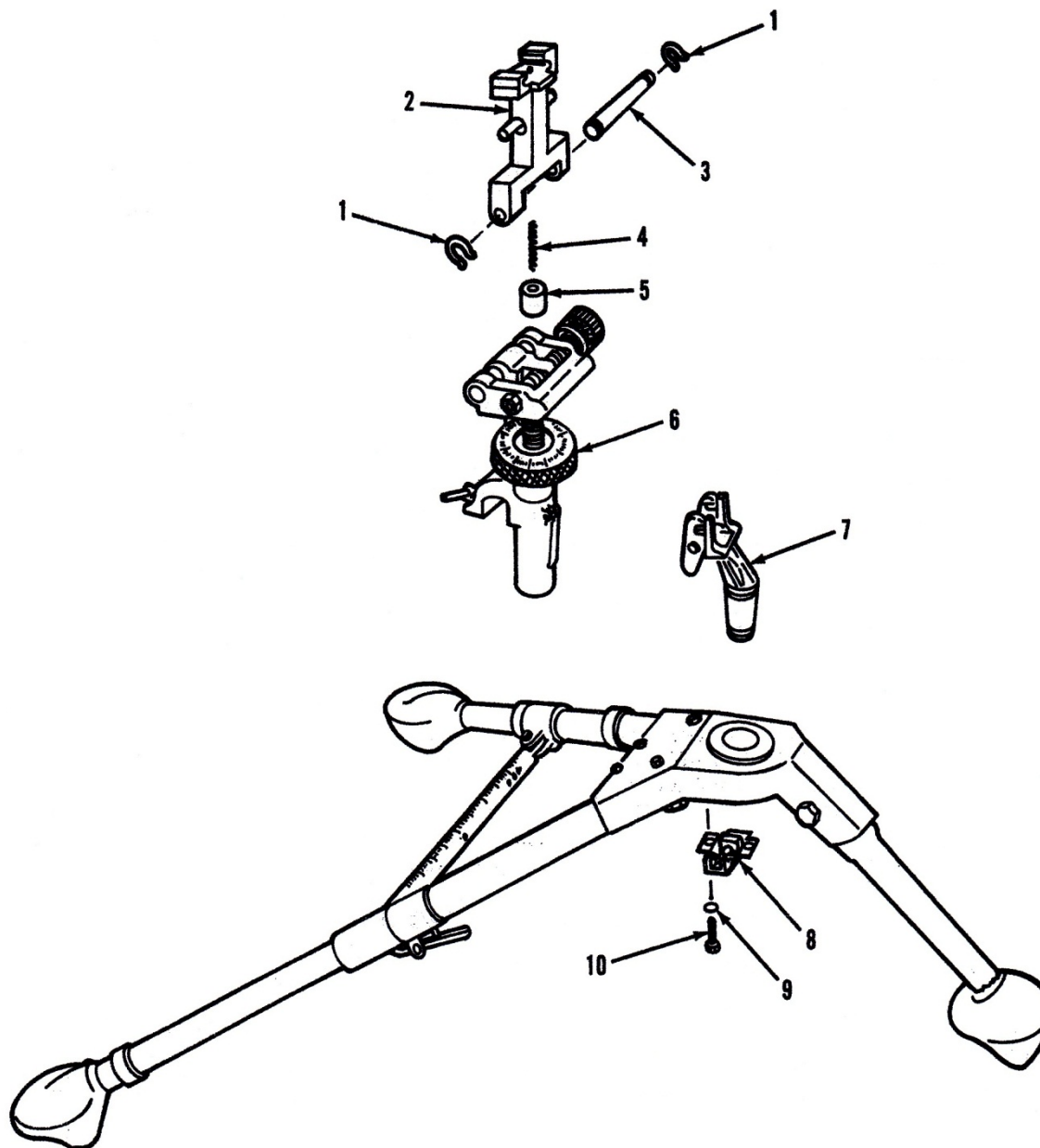
ภาพที่ 29 ขาหยังปืนกล M122 (องค์ประกอบหลัก)
