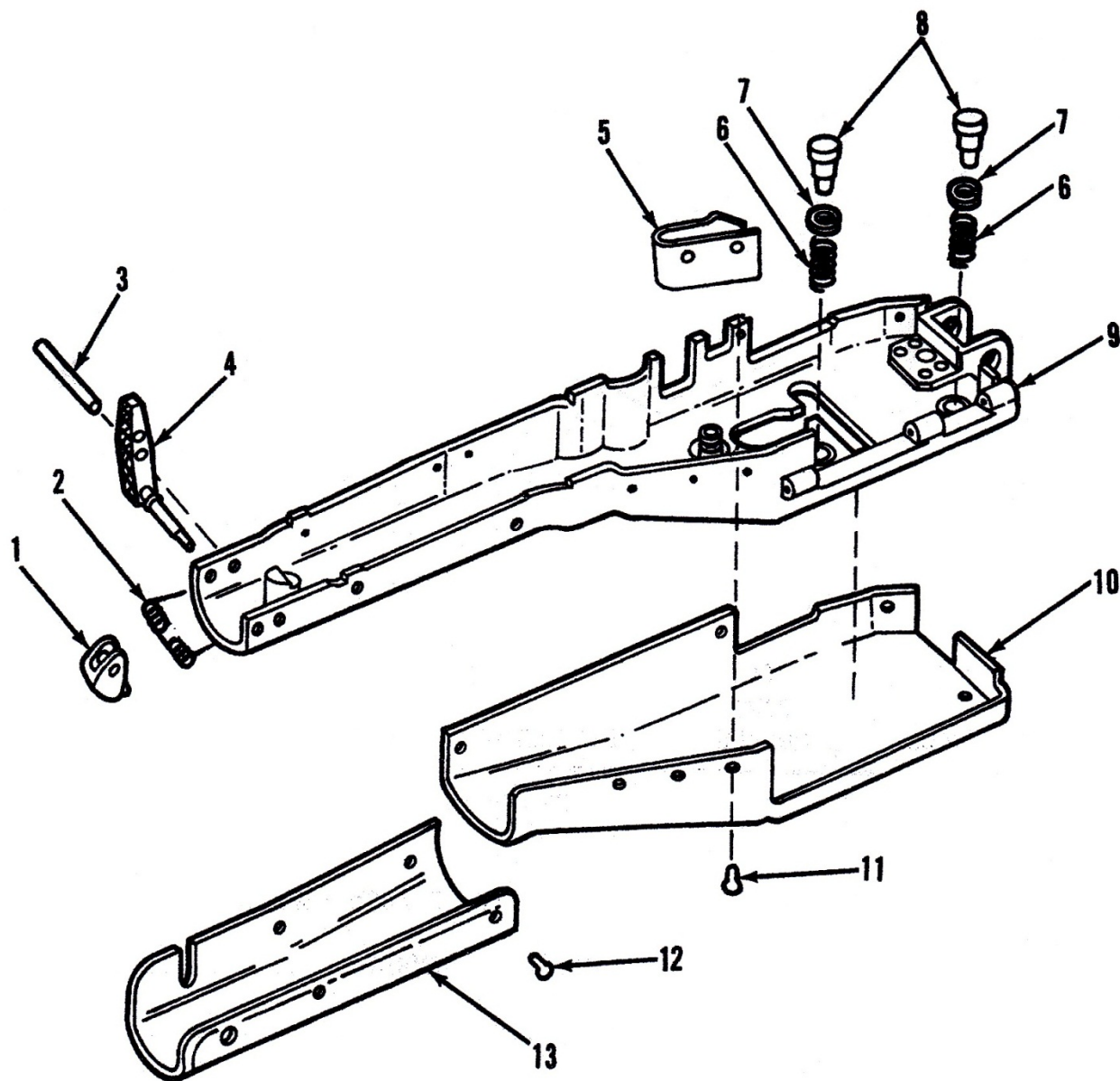
ภาพที่ 18 ชุดฝาปิดห้องลูกเลื่อน
