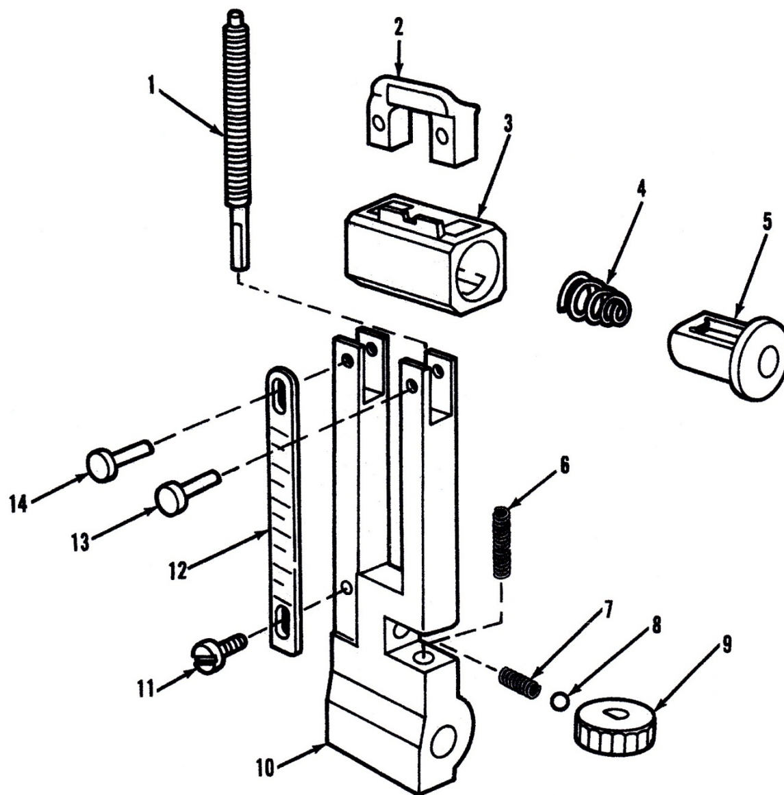
ภาพที่ 24 ชุดใบศูนย์หลัง (เฉพาะ M60)
