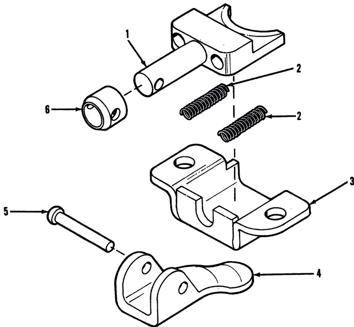
ภาพที่ 35 ชุดล็อกเดือยหัวขาหยัง
