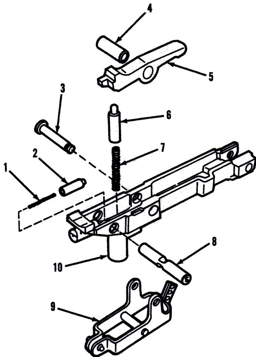
ภาพที่ 10 กระเดื่องไกและชุดเรือนห้ามไก (เฉพาะ M60D)
