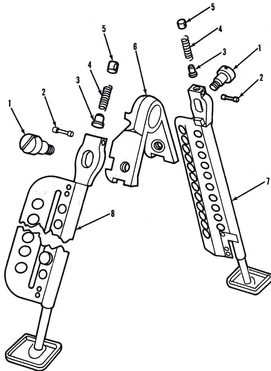
ภาพที่ 12 ขาทรายปั่นกล
