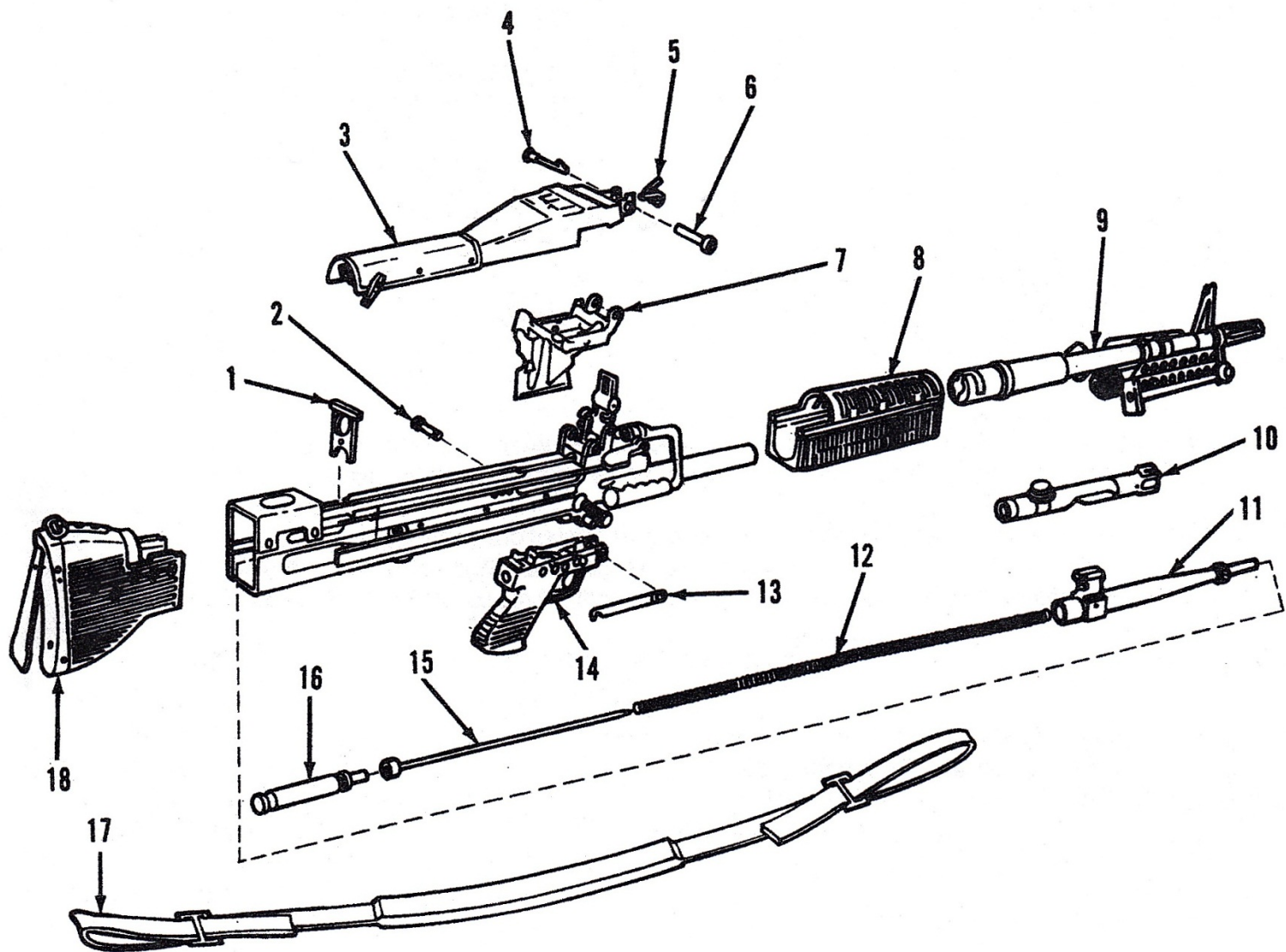
ภาพที่ 1 ปืนกล ขนาด 7.62 มิลลิเมตร M60 และ M60D (ชุดองค์ประกอบหลัก M60)
