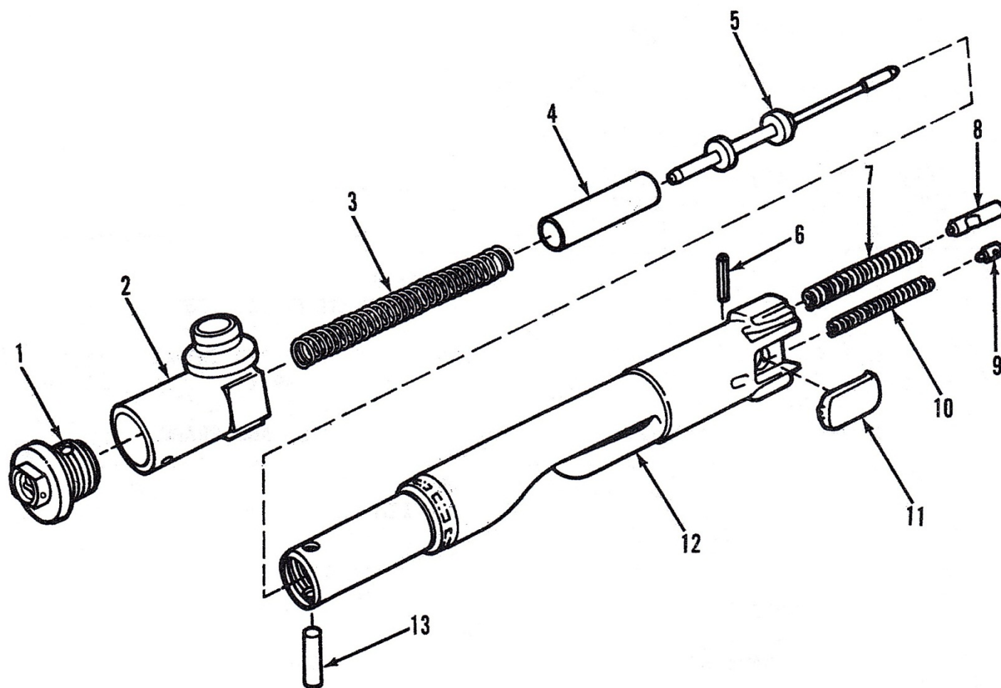
ภาพที่ 7 ชุดลูกเลื่อน
