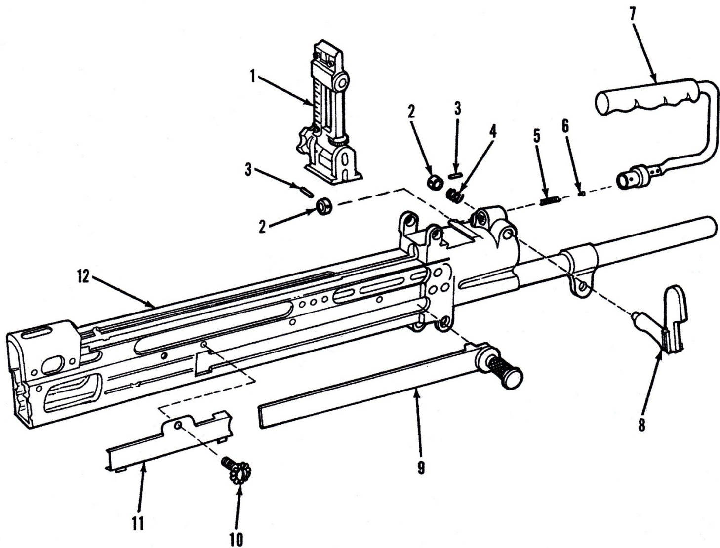
ภาพที่ 2 ปืนกล ขนาด 7.62 มิลลิเมตร M60 และ M60D (ชุดองค์ประกอบย่อย M60)
