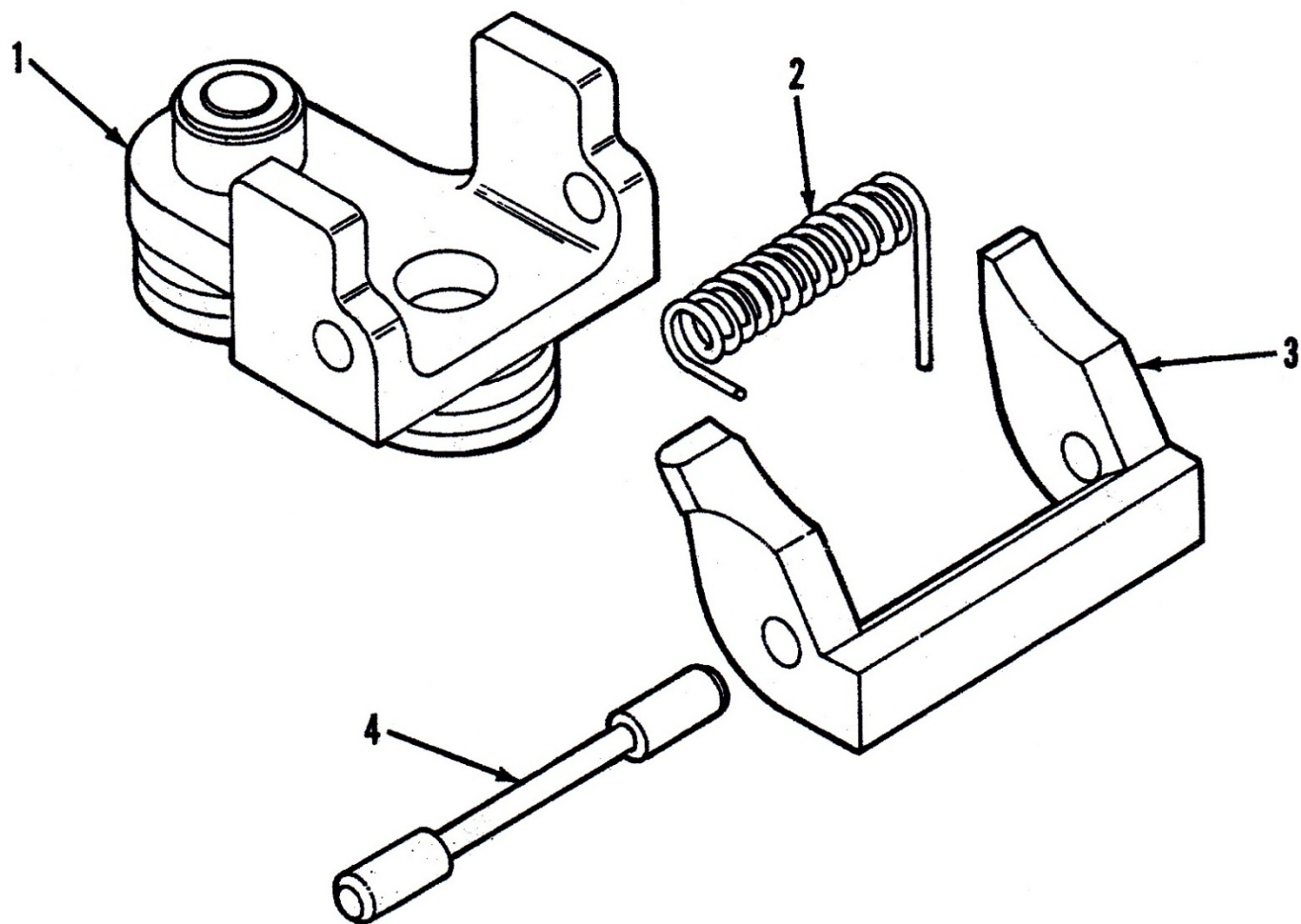
ภาพที่ 17 ชุดลั่นเลื่อนสายกระสุน
