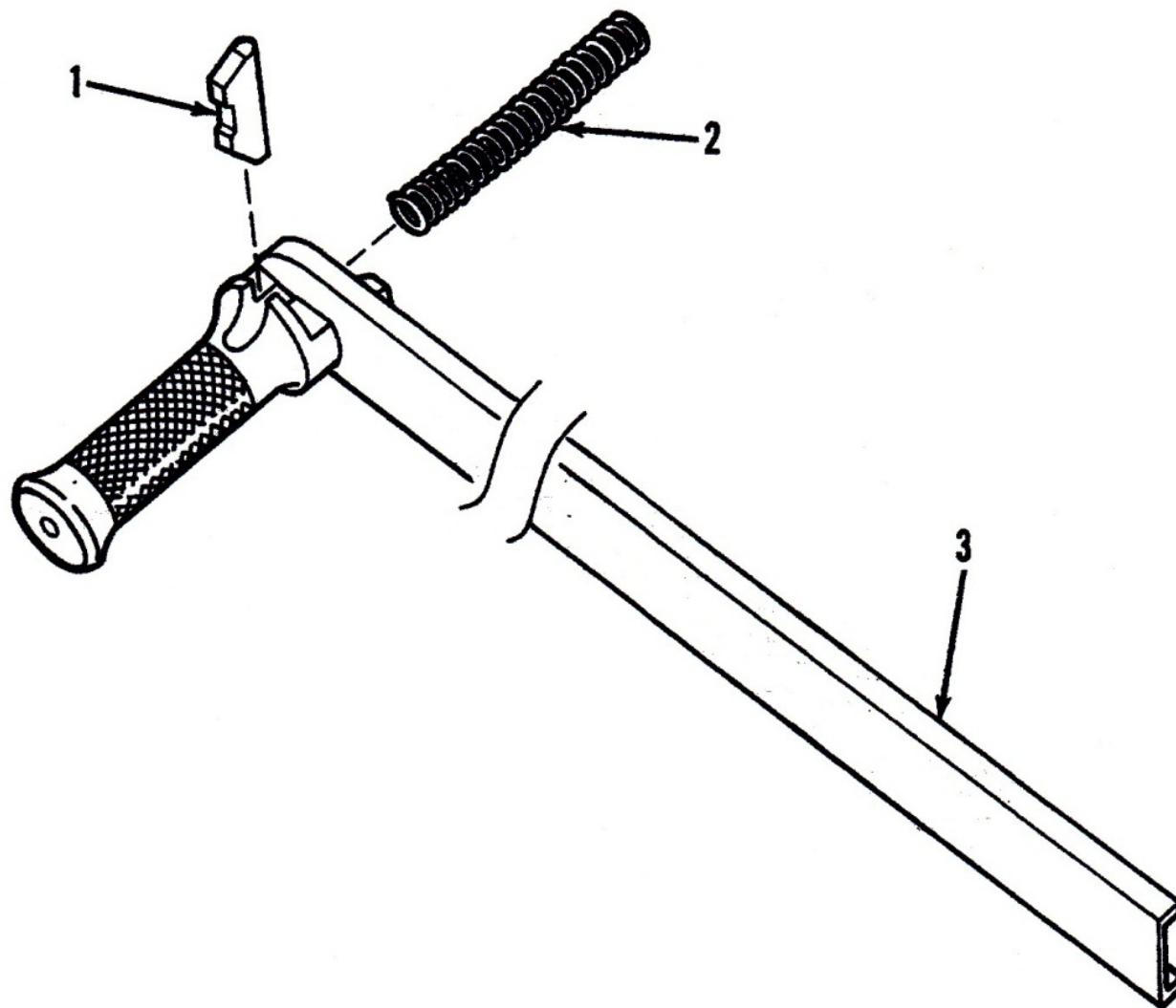
ภาพที่ 26 ชุดคันเร่งลูกเลื่อน
