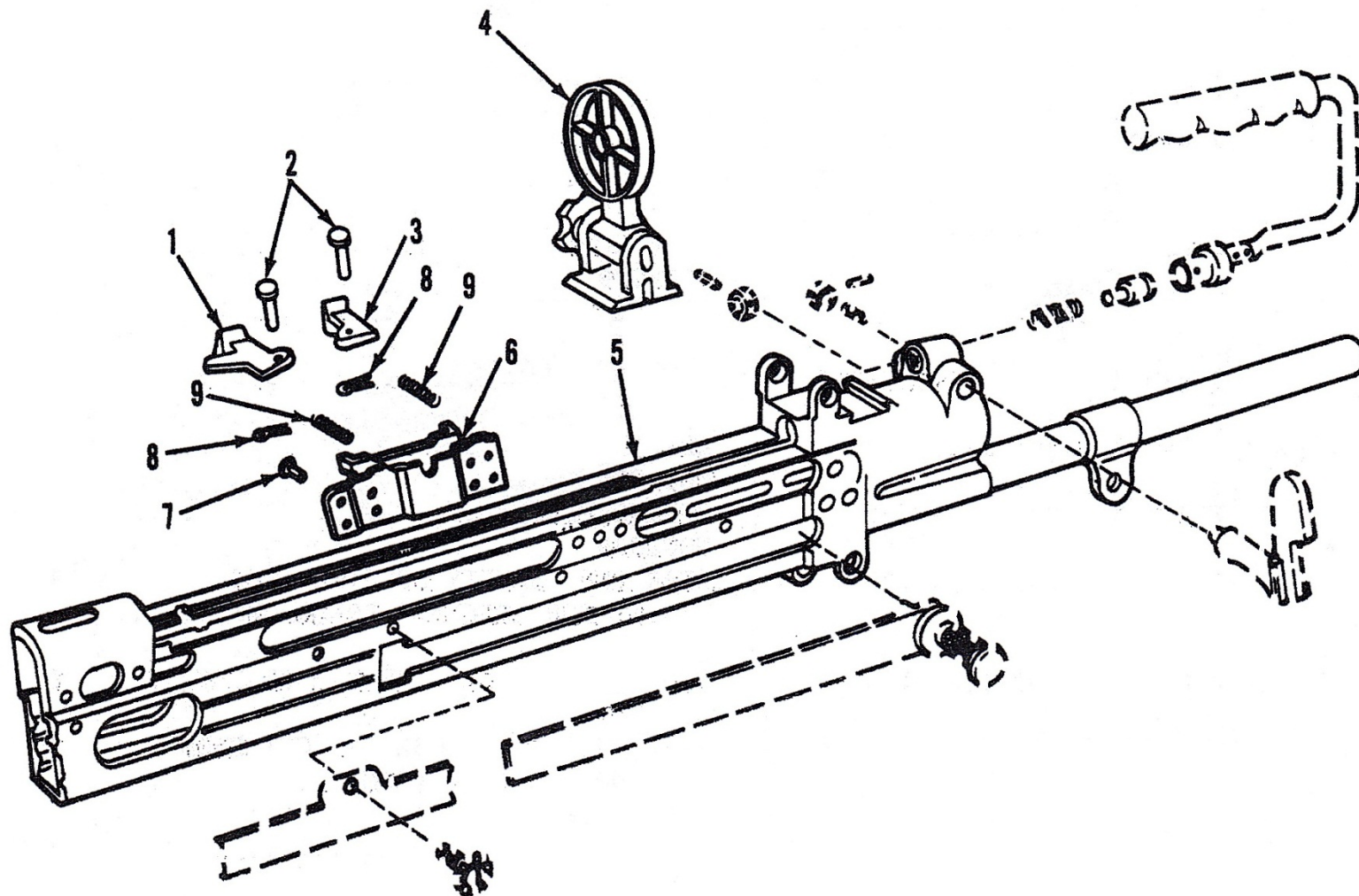
ภาพที่ 4 ปืนกล ขนาด 7.62 มิลลิเมตร M60 และ M60D (ชุดองค์ประกอบย่อย M60D)
